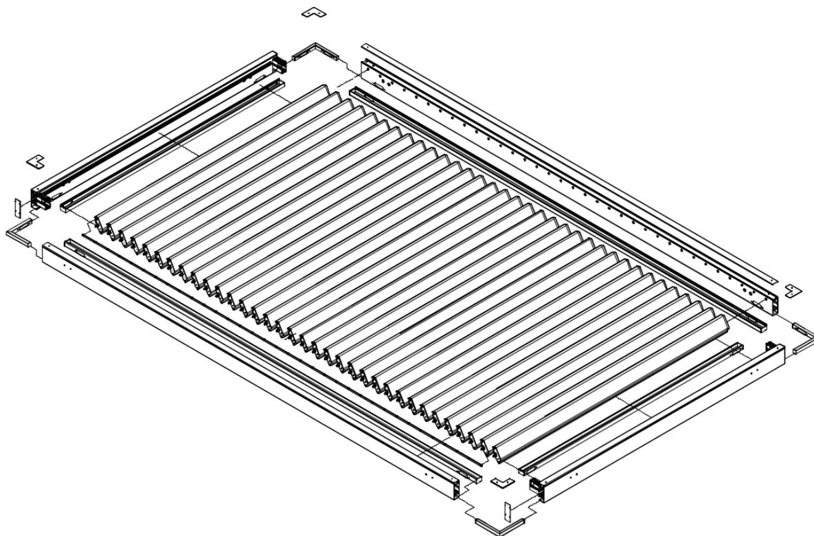
Rys. 7. Widok montażu elementów Pergoli SB400PRO R z czterema rynkami.
